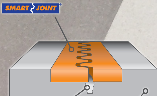
giunto degradato degraded joint pavimentazione esistente existing flooring
